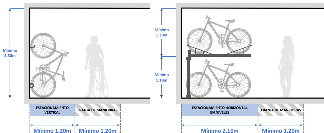
Gráfico 86: Estacionamientos de bicicletas en vertical.
