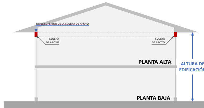
Gráfico 12: Altura en cubiertas inclinadas.
