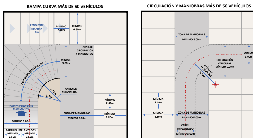
Gráfico 80: Rampas curvas y circulaciones para edificios de vivienda, comercios, oficinas y usos mixtos. Más de 50 vehículos.
