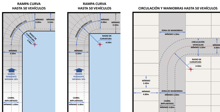
Gráfico 83: Rampas curvas y circulaciones para edificios con otros usos y para edificios de estacionamientos. Hasta 50 vehículos.
