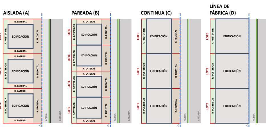
Gráfico 33: Retiros según su forma de ocupación
