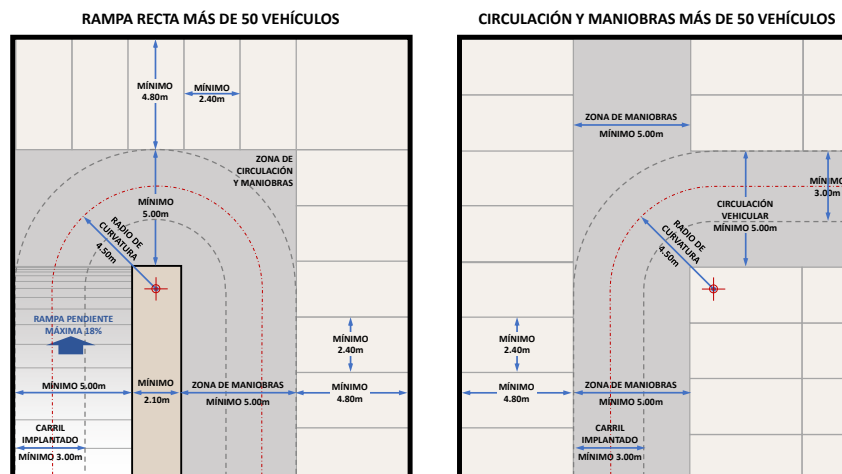
Gráfico 78: Rampas rectas y circulaciones para edificios con otros usos y para edificios de estacionamientos. Más de 50 vehículos.
