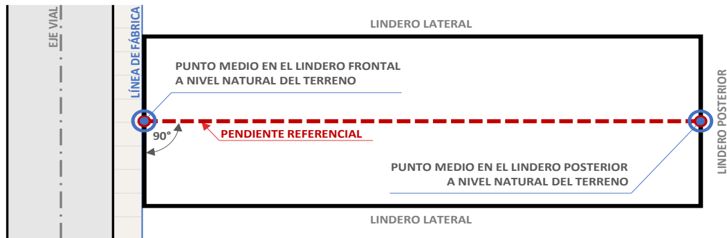
Gráfico 6: Pendiente referencial en terrenos regulares
