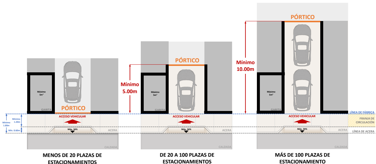
Gráfico 71: Definición de la transición de acceso a los estacionamientos
