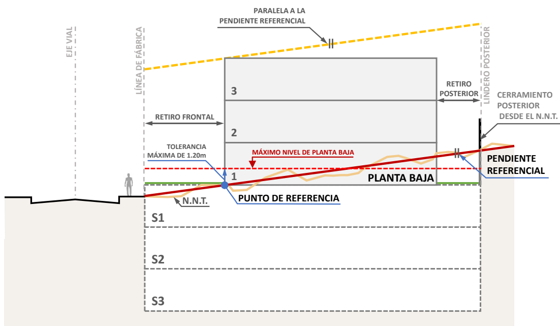
Gráfico 19: Terrenos con retiro frontal y pendiente positiva.
