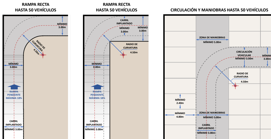
Gráfico 77: Rampas rectas y circulaciones para edificios con otros usos y para edificios de estacionamientos. Hasta de 50 vehículos.
