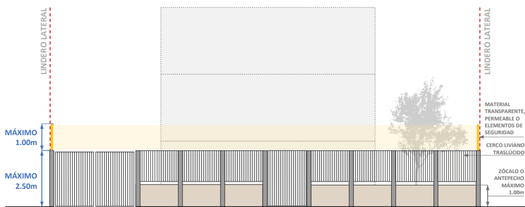
Gráfico 57: Cerramientos con muro bajo.
