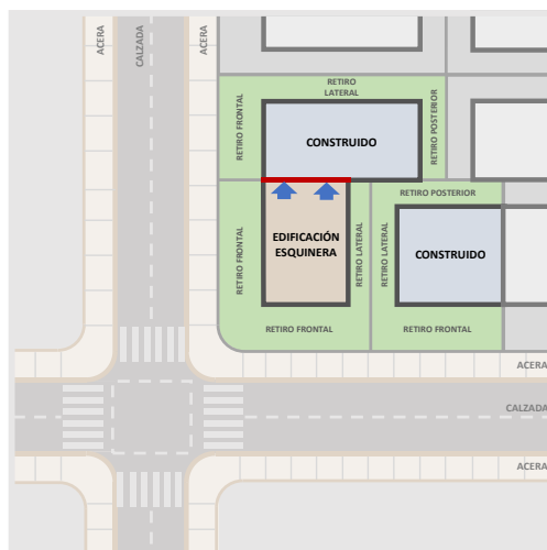
Gráfico 38: Resolución de retiro con lotes colindantes construidos y un adosado.
