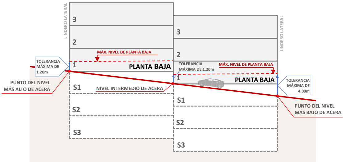
Gráfico 31: Edificaciones aterrazadas con bloques continuos en terrenos con frente menores a 30,00 metros a vías inclinadas
