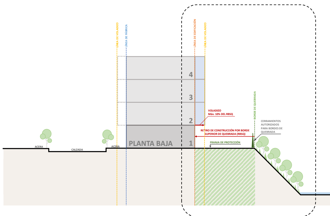
Gráfico 51: Voladizos hacia retiros de protección de quebrada y riberas de ríos.
