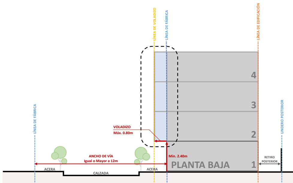
Gráfico 48: Voladizo en lotes sobre línea de fábrica y ancho de vía igual o mayor a 12,00 metros.
