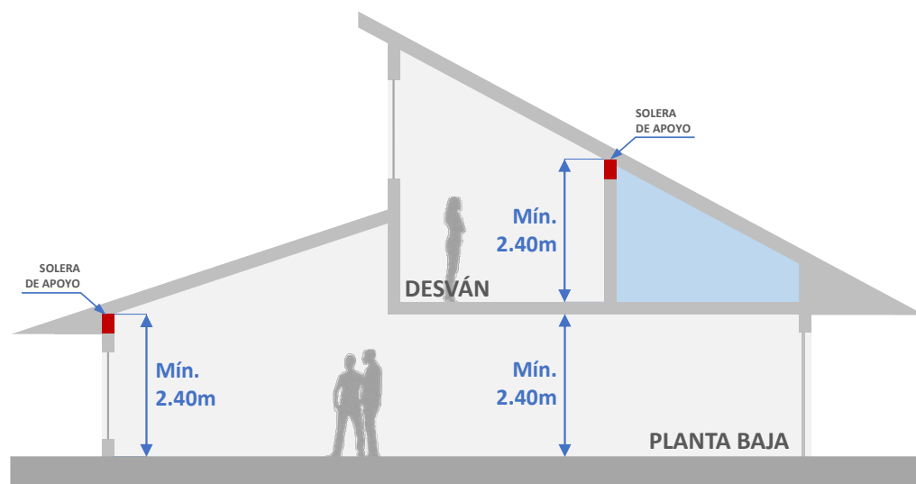
Gráfico 45: Desvanes o Buhardillas.
