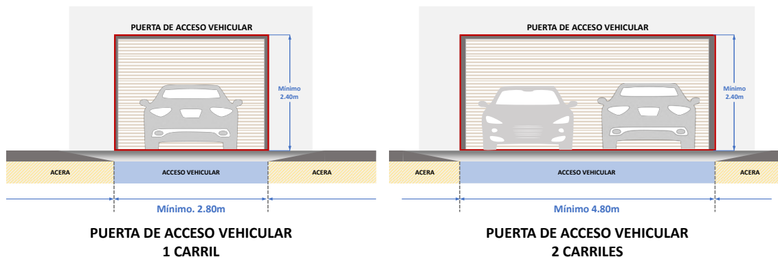
Gráfico 72: Dimensiones de ingresos vehiculares.
