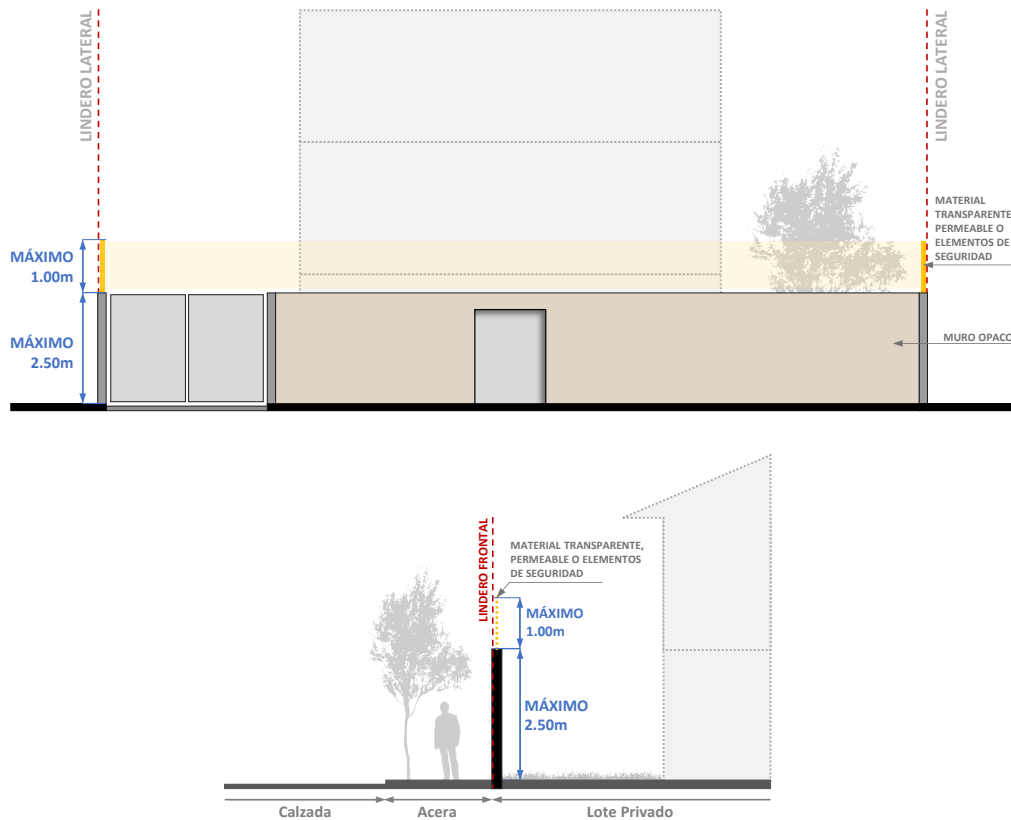
Gráfico 56: Cerramientos opacos con muro alto.
