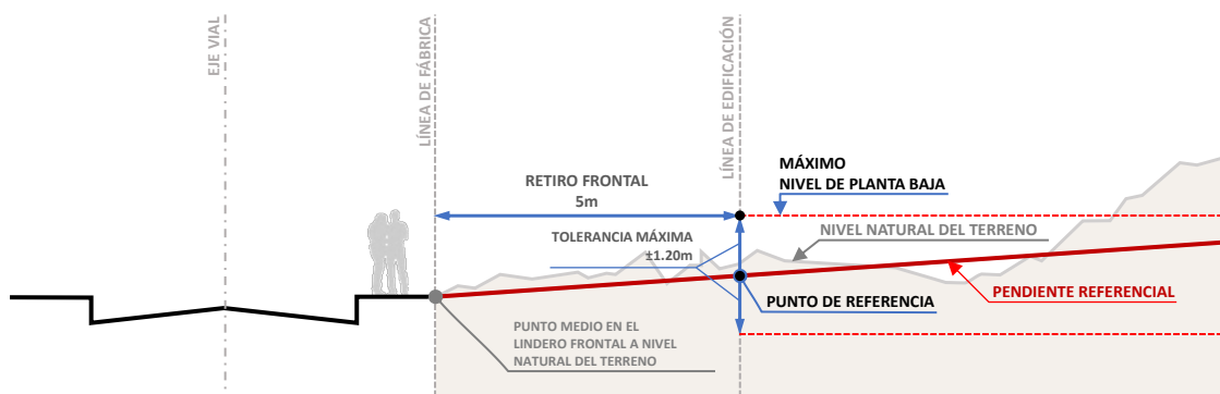
Gráfico 14: Definición de planta baja en terrenos planos con retiro frontal.
