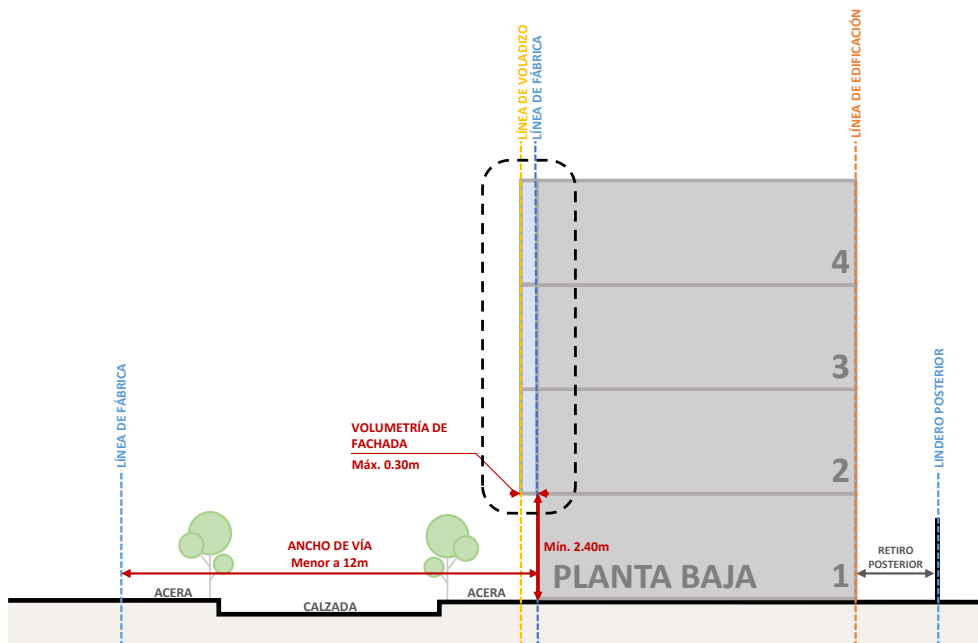
Gráfico 47: Volumetría de fachada en lotes sobre línea de fábrica y ancho de vía menor a 12,00 metros.
