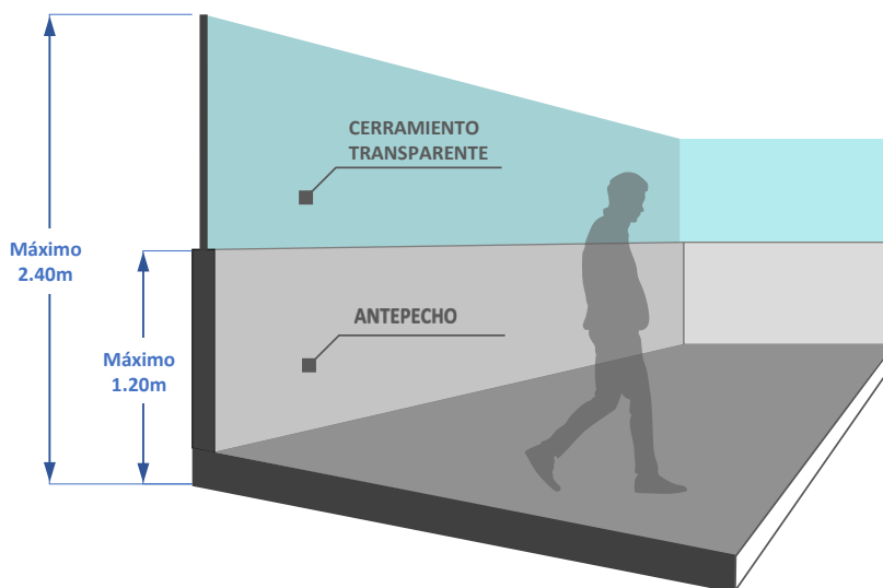
Gráfico 53: Ilustración referencial del cerramiento en terrazas.
