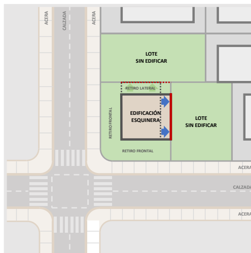
Gráfico 40: Resolución de retiro con lotes colindantes sin edificar.
