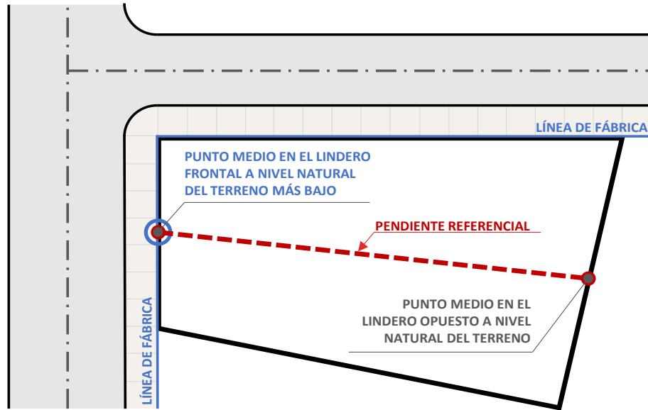
Gráfico 8: Pendiente referencial en terrenos esquineros. Ejemplo 2.
