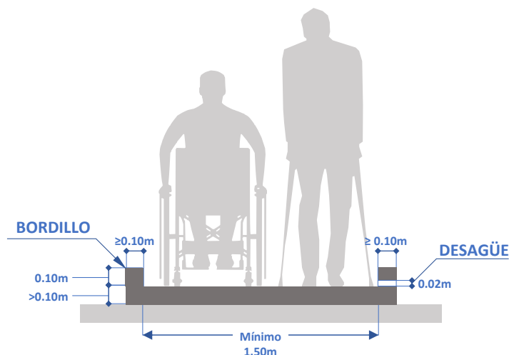
Gráfico 73: Circulaciones con desnivel
