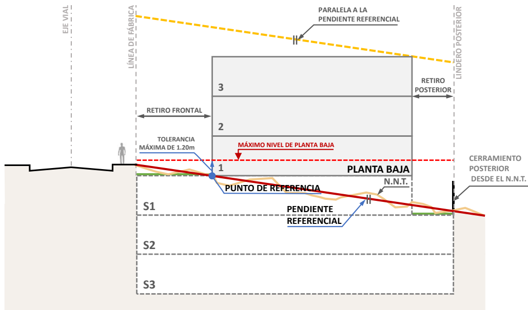
Gráfico 23: Terrenos con retiro frontal y pendiente negativa
