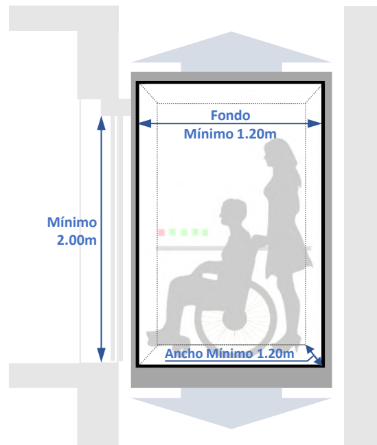
Gráfico 74: Sección en elevación de la cabina de ascensor.
