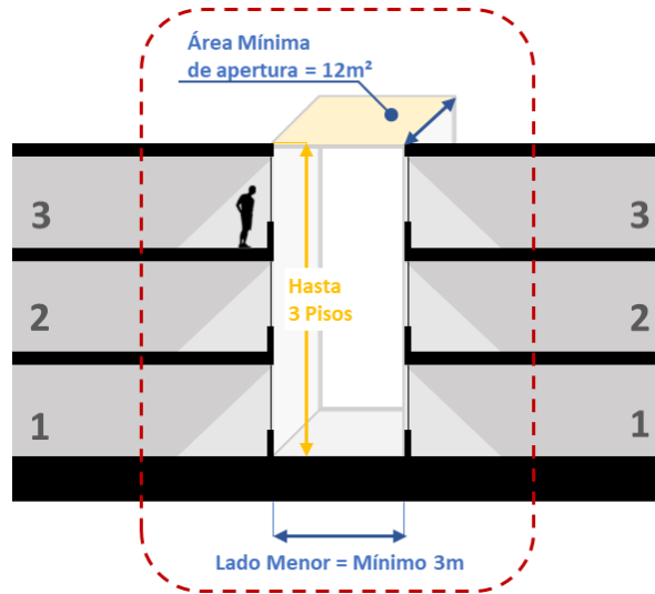
Gráfico 96: Dimensiones de los ductos de iluminación/ventilación.
