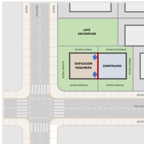
Gráfico 39: Resolución de retiro con lotes colindantes construido- adosado y lote sin edificar.
