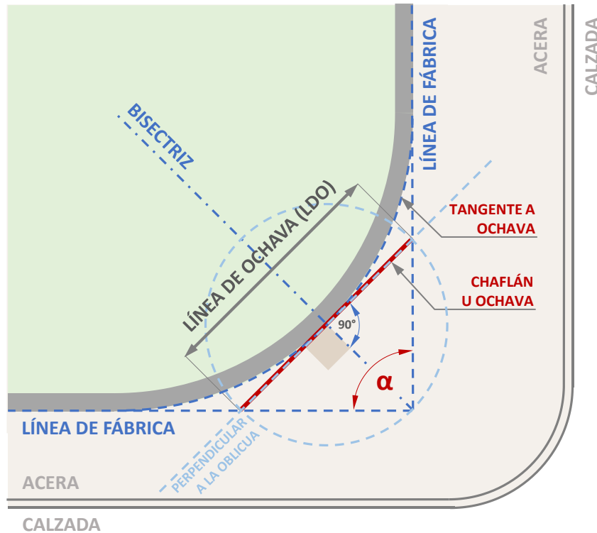
Gráfico 61: Cerramientos redondeados en lotes esquineros.
