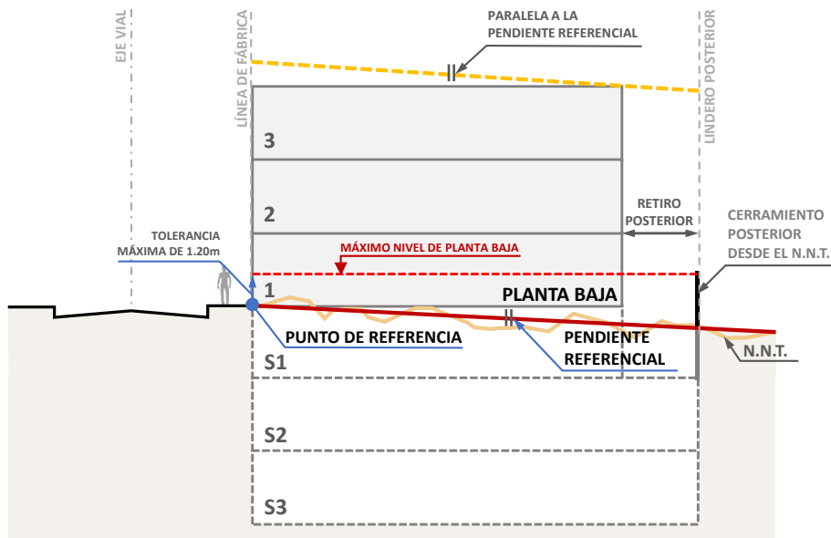
Gráfico 15: Terrenos planos sobre línea de fábrica.
