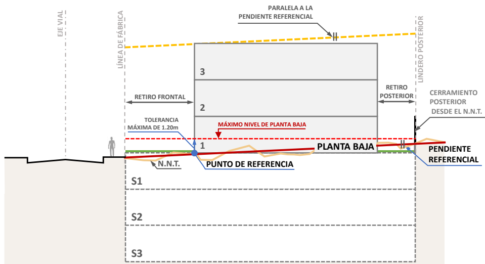
Gráfico 16: Terrenos planos con retiro frontal
