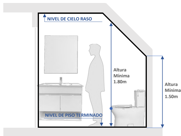
Gráfico 95: Altura mínima en baños bajo escaleras.
