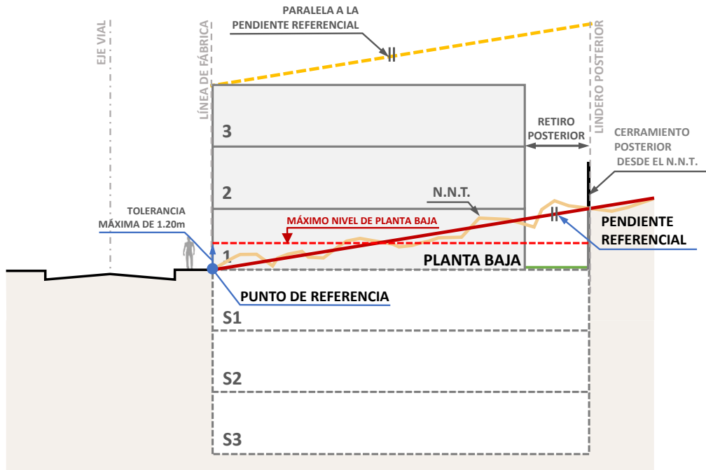
Gráfico 18: Terrenos sobre línea de fábrica y pendiente positiva.
