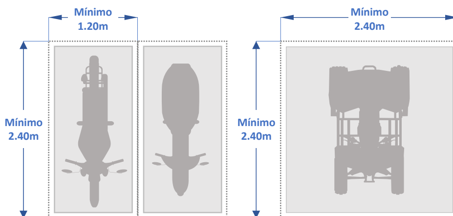
Gráfico 87: Estacionamientos para vehículos menores motorizados.
