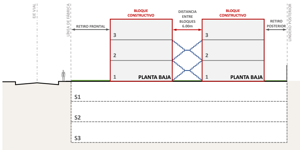
Gráfico 32: Integración entre bloques separados
