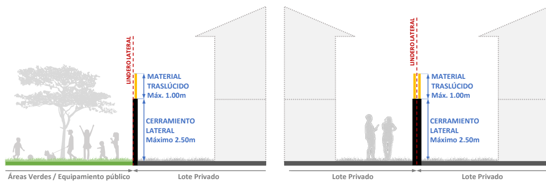
Gráfico 63: Cerramientos laterales o posteriores colindantes con áreas verdes y equipamiento público y entre lotes privados.
