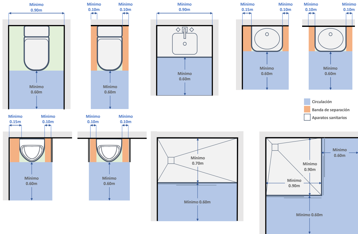
Gráfico 94: Distancias entre aparatos sanitarios.
