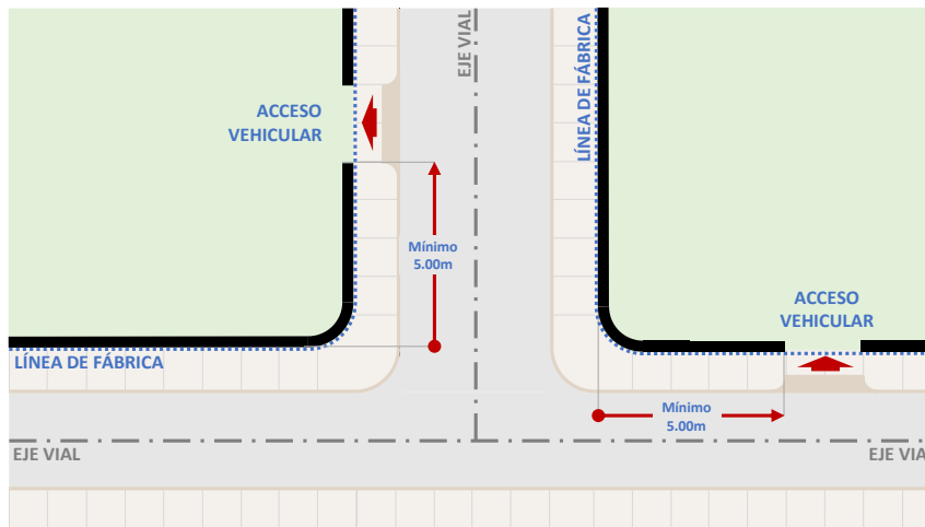
Gráfico 68: Ingresos vehiculares en lotes esquineros.
