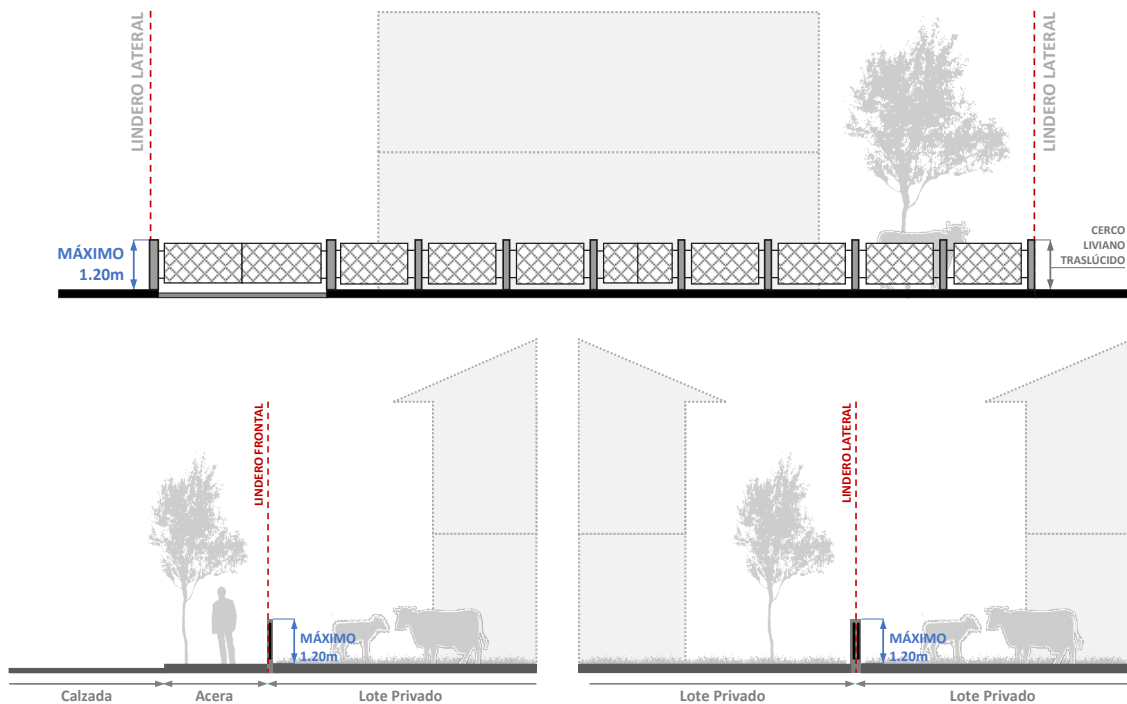
Gráfico 59: Cerramientos livianos o rural.
