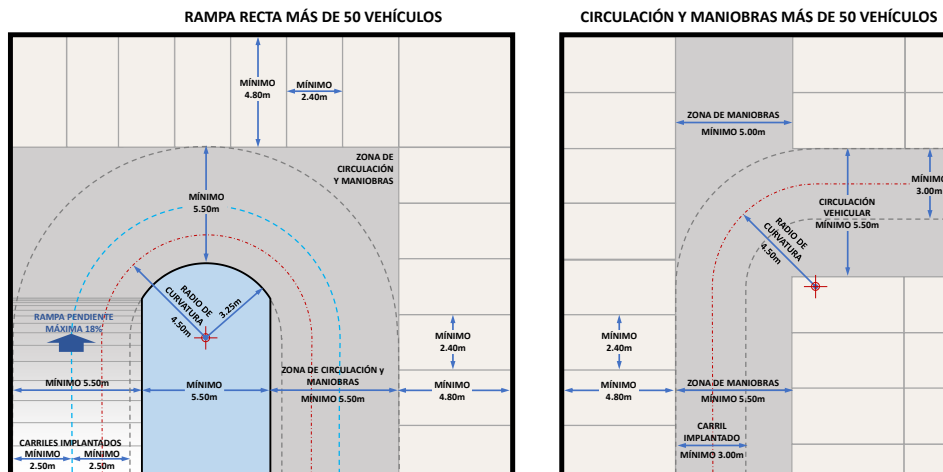
Gráfico 82: Rampas rectas y circulaciones para edificios con otros usos y para edificios de estacionamientos. Más de 50 vehículos.
