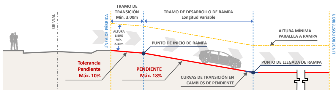
Gráfico 76: Accesos de rampas vehiculares descendientes en terrenos en formas de ocupación Sobre línea de fábrica (D).
