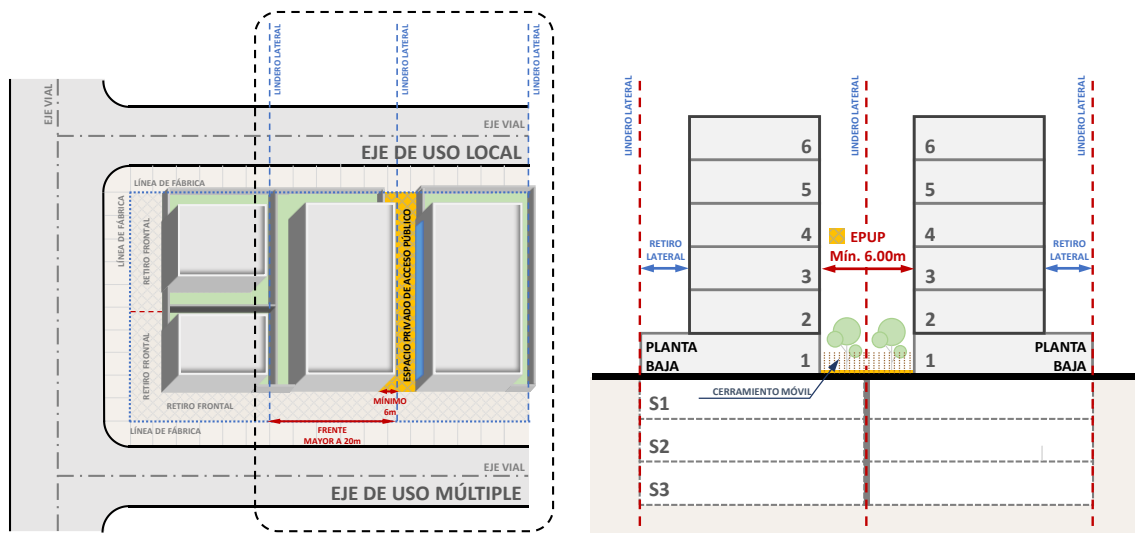
Gráfico 34: Integración del retiro lateral.
