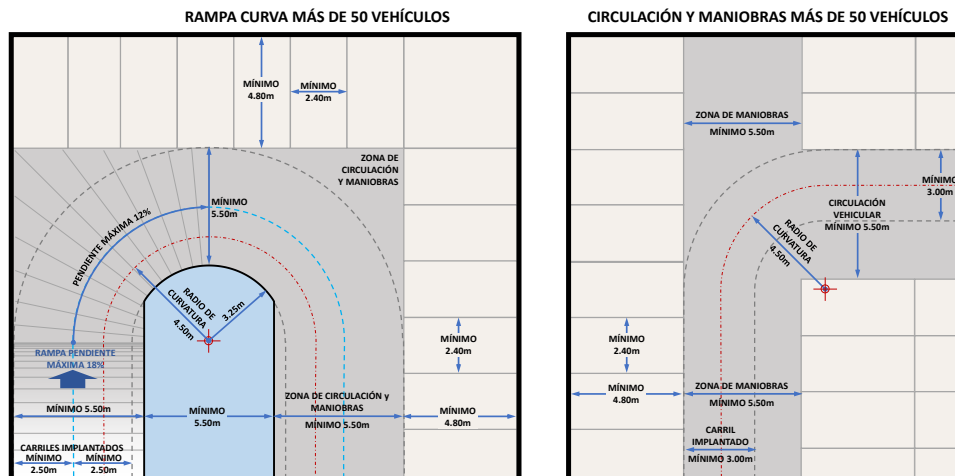
Gráfico 84: Rampas curvas y circulaciones para edificios con otros usos y para edificios de estacionamientos. Más de 50 vehículos.
