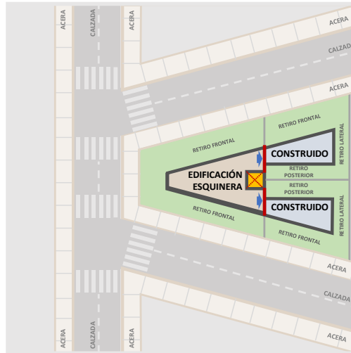
Gráfico 41: Resolución de retiro con pozos de iluminación- ocupación pareada (B).
