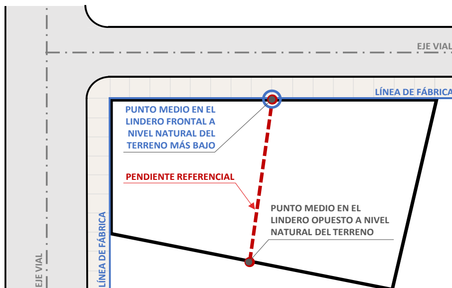
Gráfico 7: Pendiente referencial en terrenos esquineros. Ejemplo 1.
