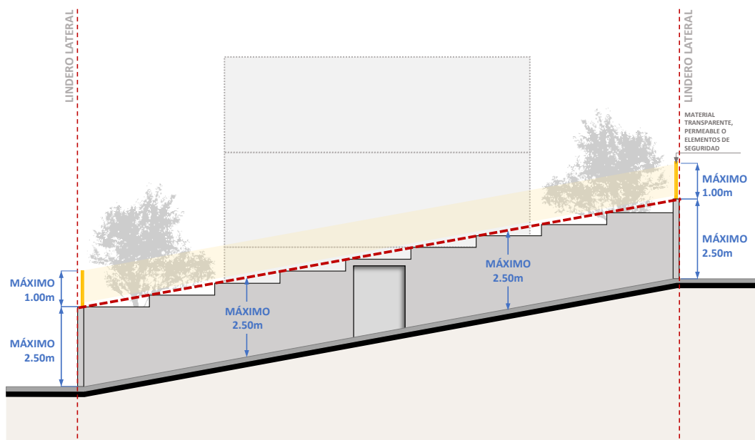
Gráfico 55: Cerramientos en pendiente.
