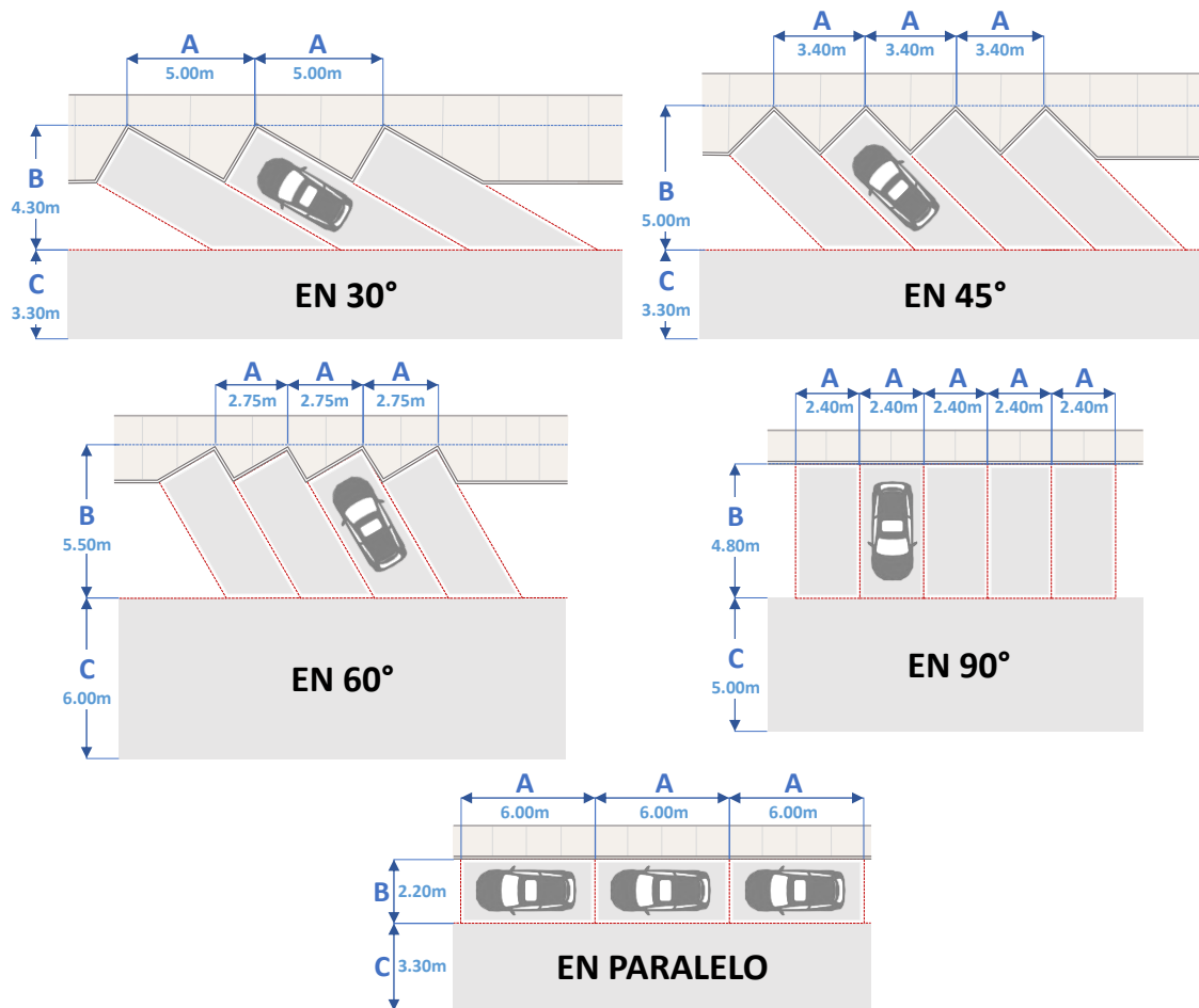
Gráfico 89: Formas de colocación de puestos de estacionamiento.
