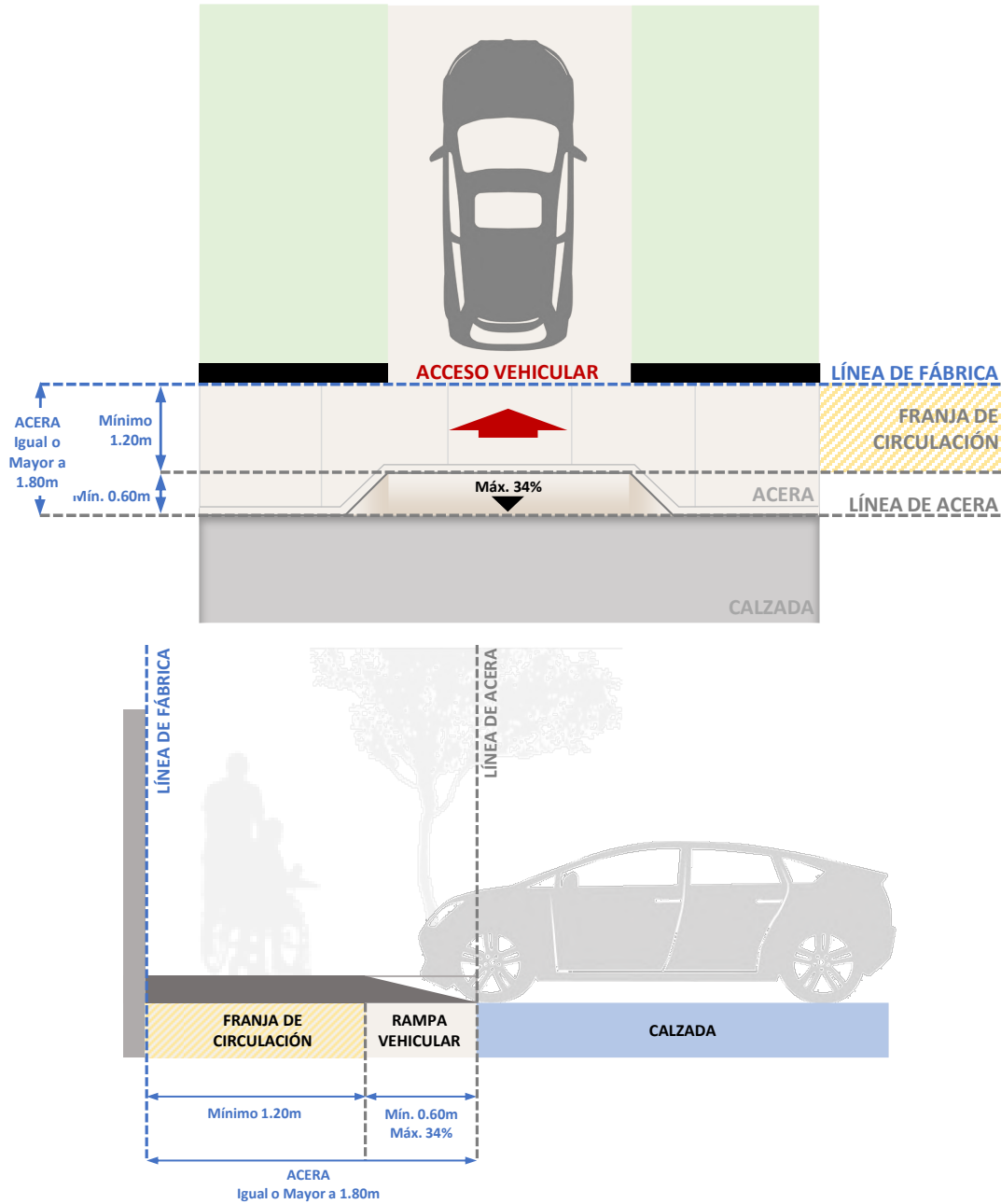
Gráfico 69: Ingresos vehiculares en aceras mayores a 1,80 metros.
