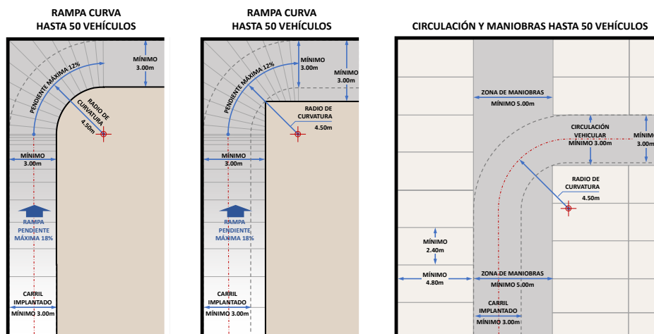
Gráfico 79: Rampas curvas y circulaciones para edificios de vivienda, comercios, oficinas y usos mixtos. Hasta 50 vehículos.
