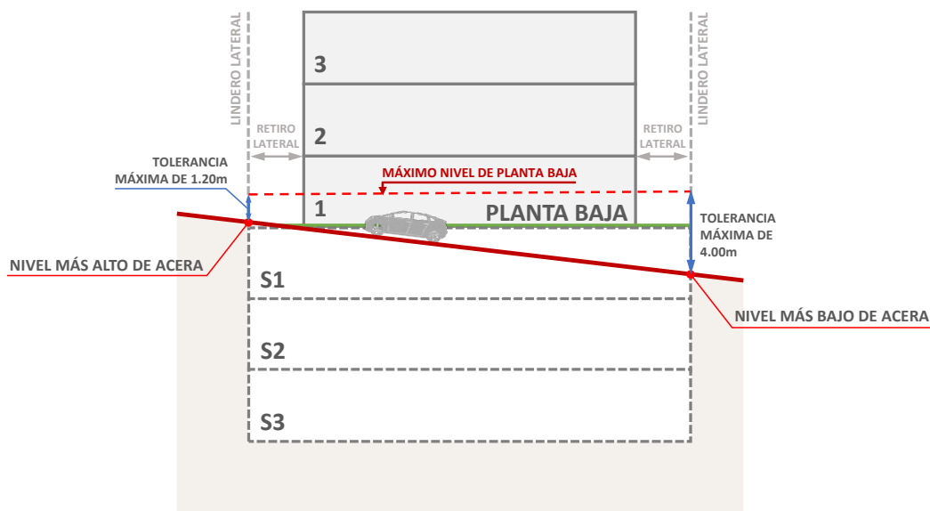
Gráfico 26: Terreno con frente a vías inclinadas con retiros laterales
