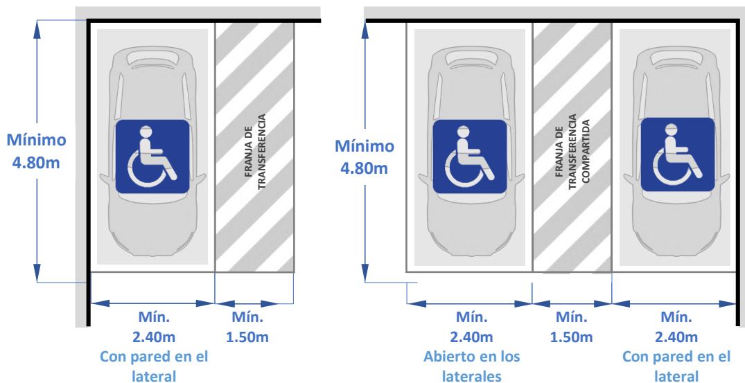
Gráfico 91: Estacionamientos para vehículos livianos de personas con movilidad reducida
