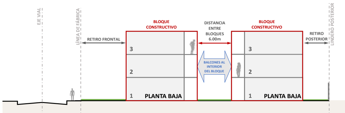
Gráfico 52: Balcones en edificaciones entre bloques.
