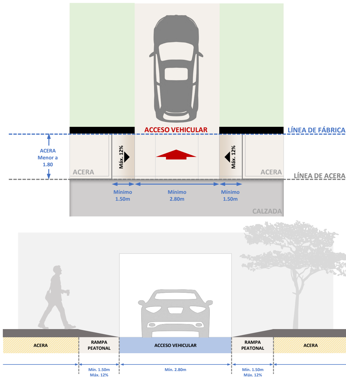
Gráfico 70: Ingresos vehiculares en aceras menores a 1,80 metros.
