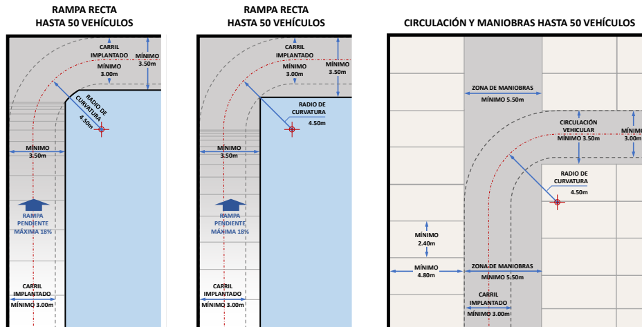
Gráfico 81: Rampa recta y circulaciones para edificios con otros usos y para edificios de estacionamientos. Hasta 50 vehículos.
