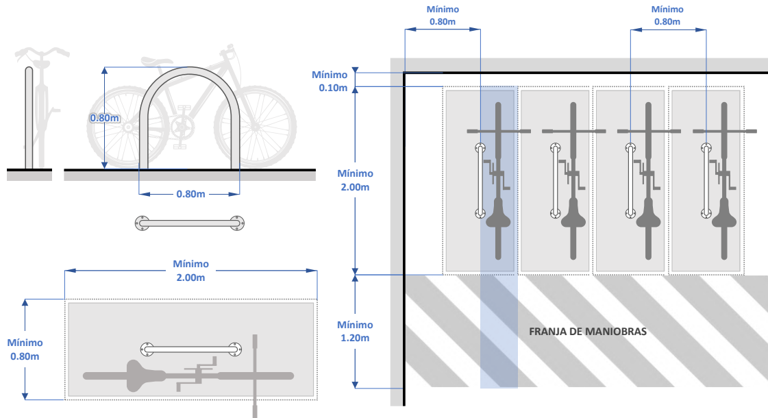
Gráfico 85: Estacionamientos para vehículos menores no motorizados.
