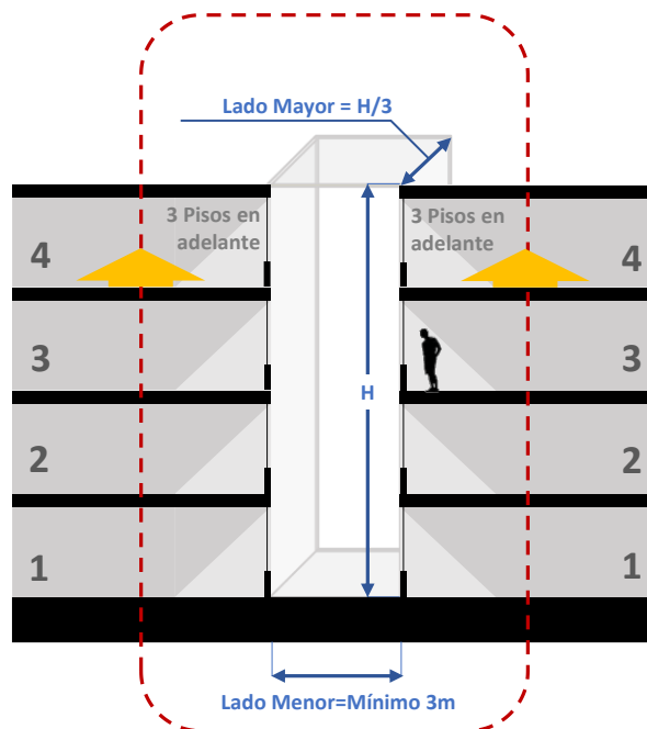
Gráfico 97: Dimensiones de los ductos de iluminación/ventilación.
