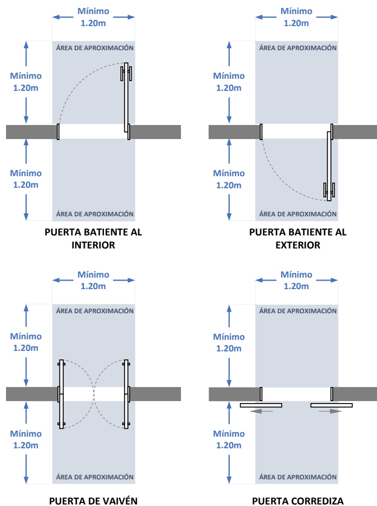
Gráfico 64: Área de aproximación en puertas de ingreso.
