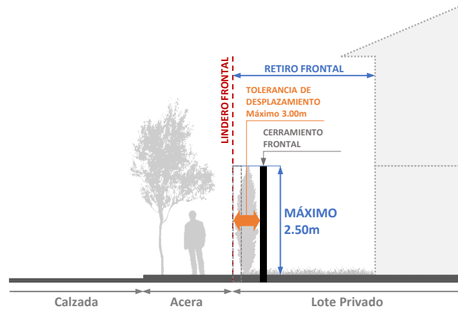
Gráfico 60: Cerramientos en retiros frontales.
