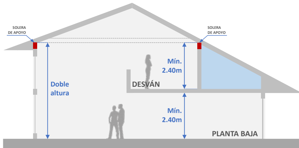
Gráfico 46: Espacios habitables de doble altura.
