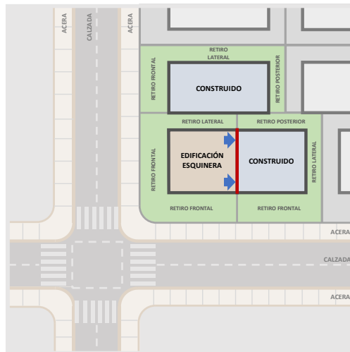
Gráfico 37: Resolución de retiro con lotes colindantes construidos y adosados.
