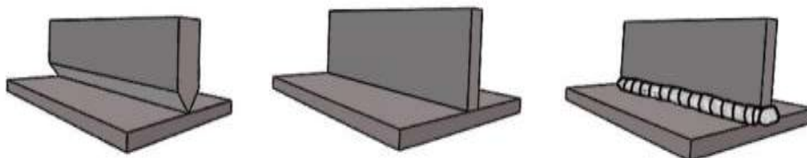
Figura 125: Juntas en T
