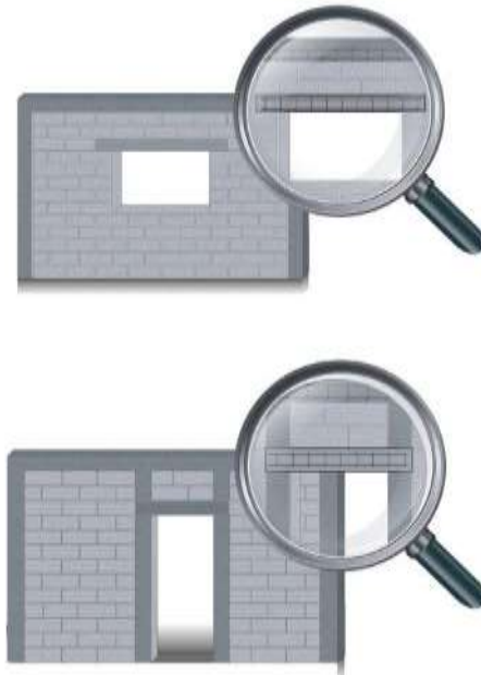
Figura 72: Dinteles alrededor de puertas y ventanas
