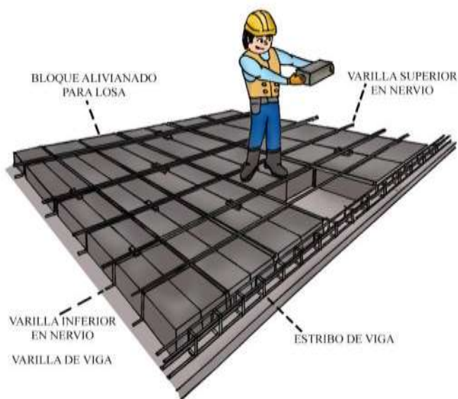
Figura 92: Colocación de bloques alivianados en la losa
