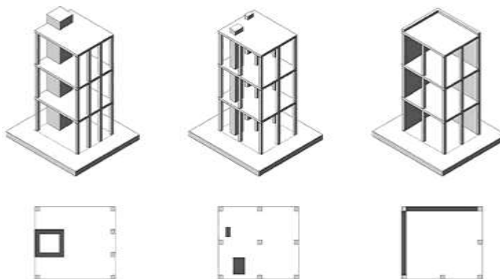
Figura 10: Centro de rigidez no coincide con centro de masa
