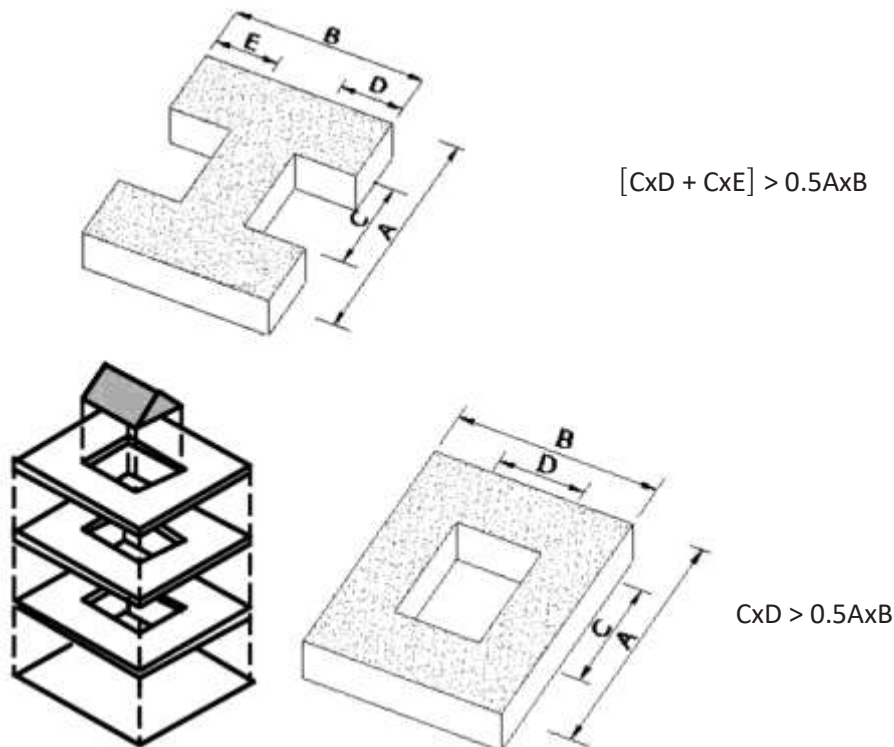
Figura 8: Discontinuidades en el sistema de piso
