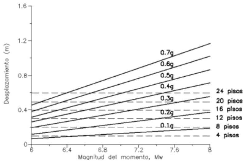
Figura 67: Comparación del máximo desplazamiento espectral elástico para el 5% de amortiguamiento en función del PGA y la magnitud del momento con R.C. Desplazamientos de fluencia del pórtico.
