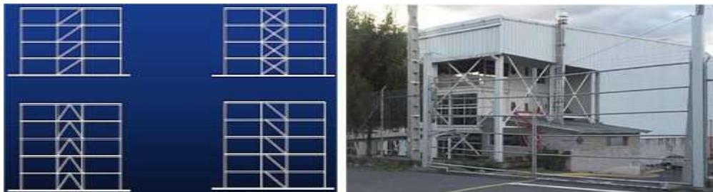
Figura 122: Tipo de sistema estructural: Pórtico de acero laminado con diagonales (S2).
