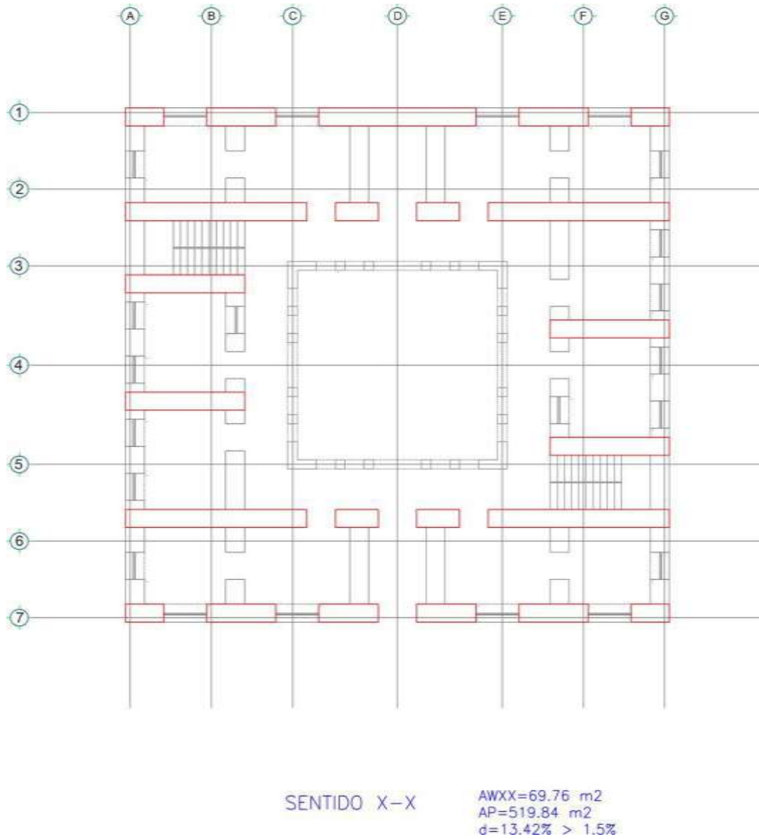
Figura 91: Configuración estructural y densidad de muros en planta sentido X-X
