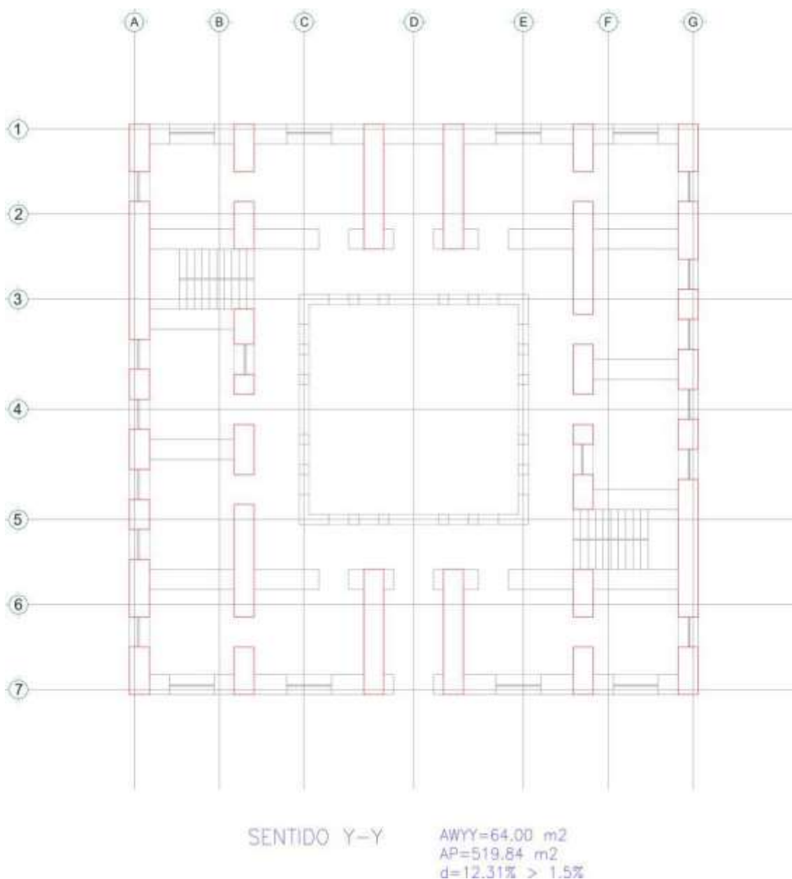
Figura 92: Configuración estructural y densidad de muros en planta sentido Y-Y
