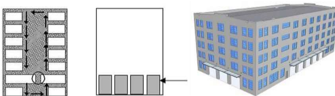
Figura 131: Irregularidad vertical: Piso débil
