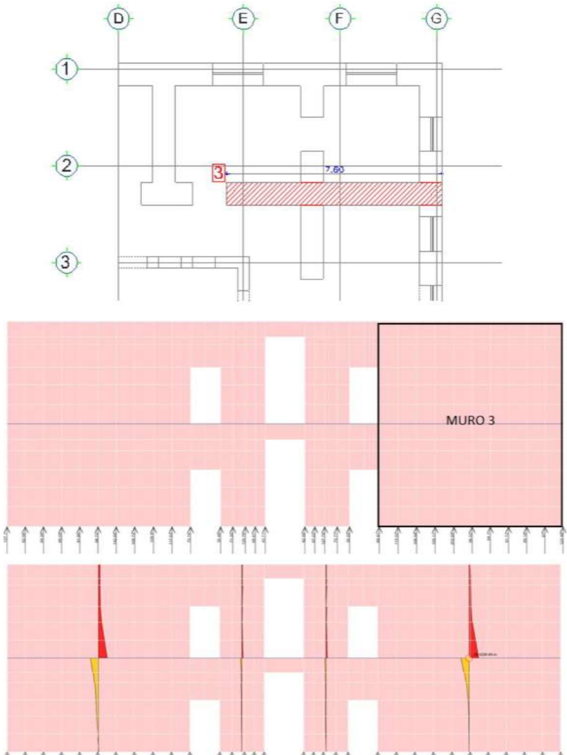
Figura 97: Resultados de diseño Muro 3
