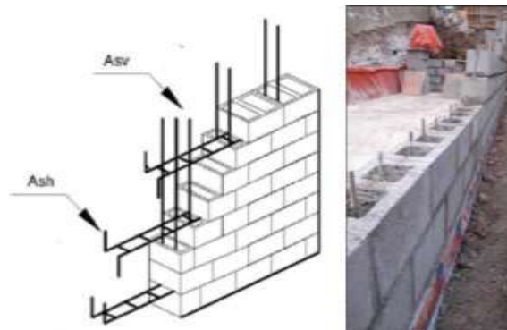
Figura 115: Tipo de sistema estructural: Mampostería reforzada (RM).
