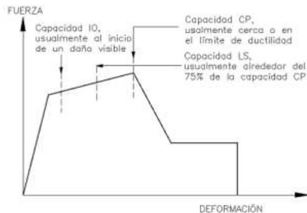
Figura 57: Criterios de Aceptación según ASCE 41
