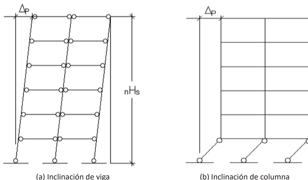
Figura 65: Mecanismos de respuesta inelástica en pórticos
