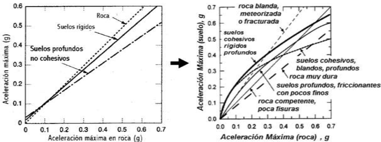
Figura 36: Relación aproximada entre la aceleración pico en roca y otros tipos de condiciones locales de sitio, propuesta por Seed et al., 1976 (figura izquierda) y modificado de Seed et al, 1997 (figura derecha)
