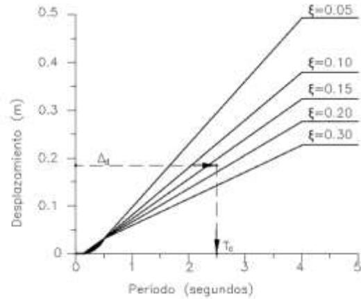
(d) Espectro de desplazamiento de diseño
