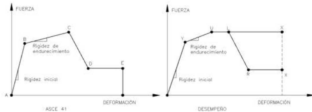
Figura 56: Modelos prácticos para estudiar el comportamiento histerético
