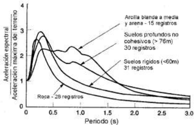
Figura 37: Espectros de respuesta medio normalizados (5% amortiguamiento) para diferentes condiciones locales de sitio. (Seed et al.,1976)
