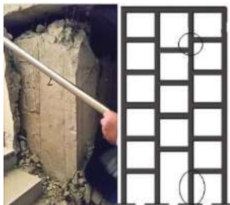
Figura 23: Columnas cortas o esbeltas: losas en niveles intermedios
