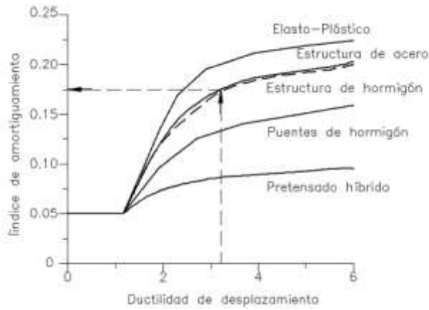
(c) Amortiguamiento equivalente vs. Ductilidad
