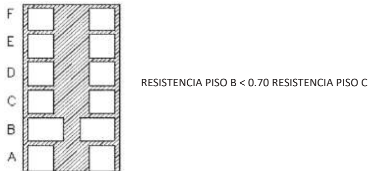
Figura 20: Discontinuidad en la resistencia
