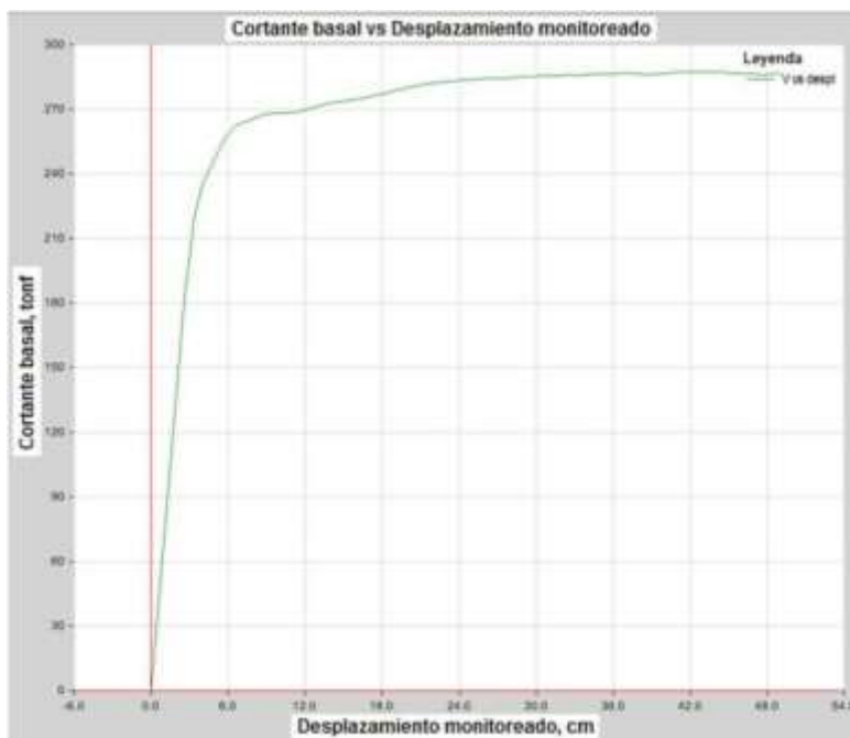
Figura 50: Curva de Capacidad
