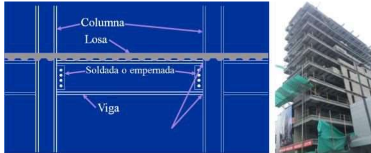
Figura 121: Tipo de sistema estructural: Pórtico de acero laminado (S1).
