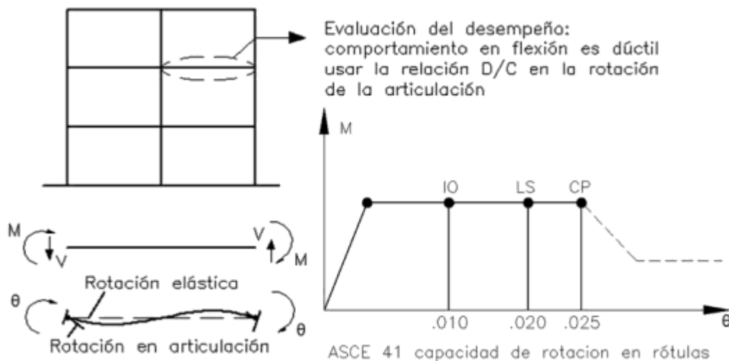
Figura 59: Diagrama Momento Curvatura para el Hormigón
