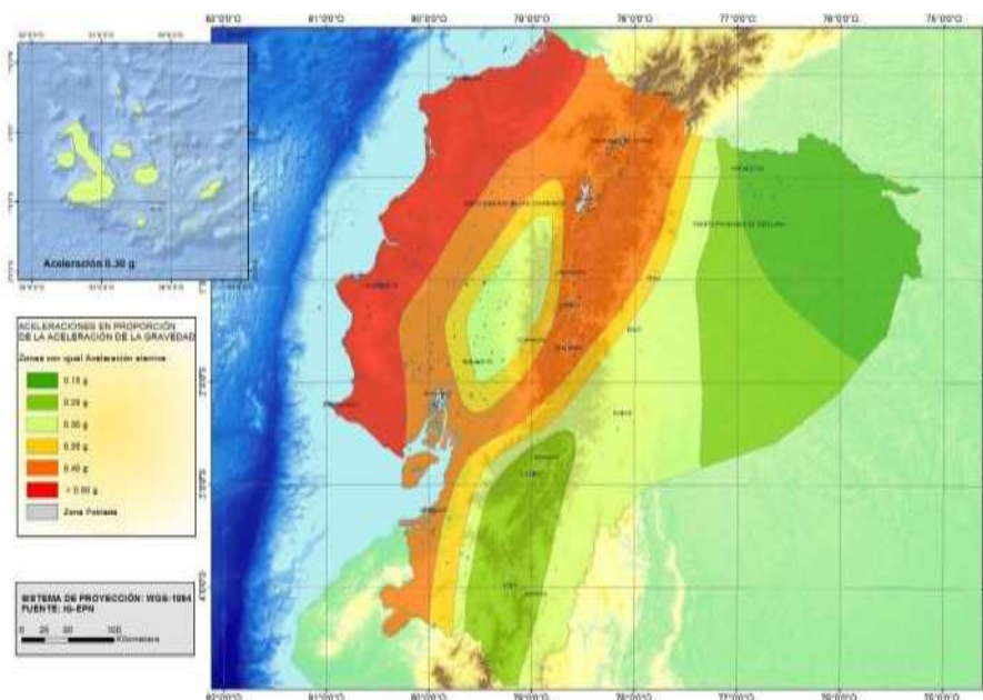
Figura 86: Zonas sísmicas para propósitos de diseño
