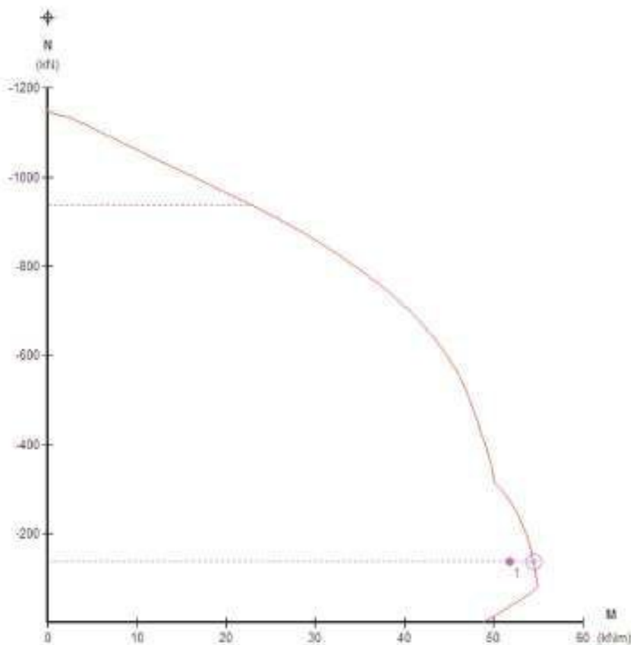
Figura 31: Diagrama de Interacción de la Columna Analizada
