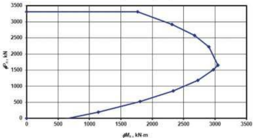
Diagrama de Interacción Carga Axial - Momento NEC-SE-MP - Diseño por Resistencia LRFD f'_m = 8 \text{ MPA} , L=4000 \text{ mm} , long, e= 20 \text{ cm} , columnas con 4\phi 12 \text{ mm} en los extremos Incluye esbeltez por Cargas Axiales
